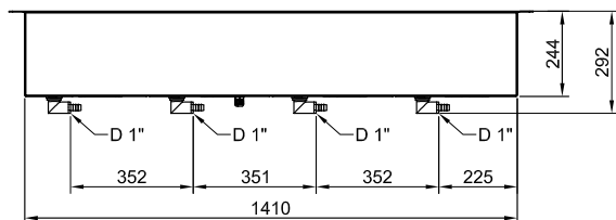
Boční
